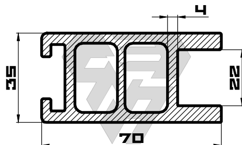
ИЗАР-А076 m=2704 (г/л.м)
