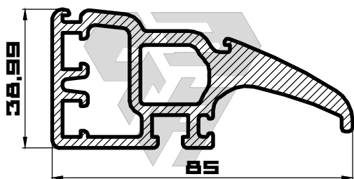
ИЗАР-АD37 m=2775 (гp/n.м)
