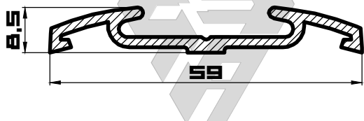
ИЗАР-А079 m=477 (г/л.м)
