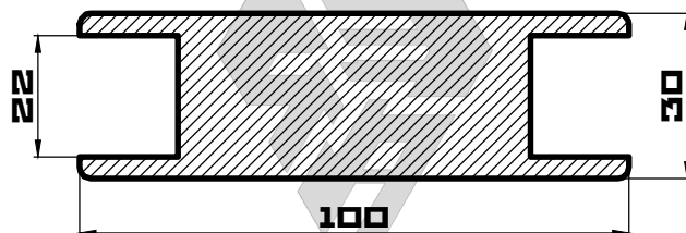
ИЗАР-АD60 m=5975 (гp/n.м)
