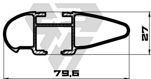
ИЗАР-А013 m=800 (гp/n.m)
