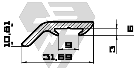
ИЗАР-AD54 m=311 (гг/н.м)
