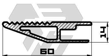
ИЗА-А021 m=846 (гp/н.м)
