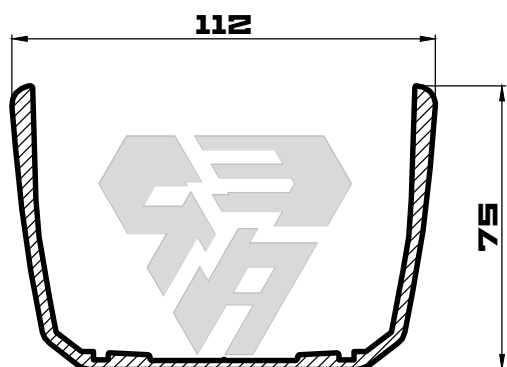
ИЗА-А023 m=2323 (гp/н.м)
