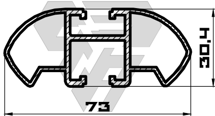
ИЗА-А017 m=1136 (гp/н.м)
