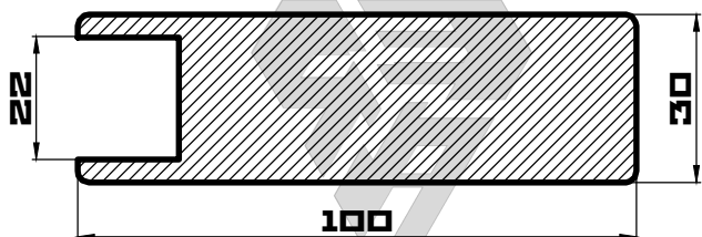
ИЗАР-АD61 m=7047 (гp/n.м)
