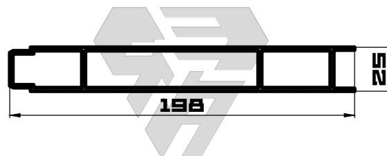
ИЗА-А088 m=2358 (гp/n.m)
