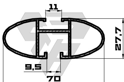
ИЗАР-А015 m=795 (гp/n.m)
