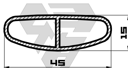
ИЗА-А086 m=453 (гp/n.m)
