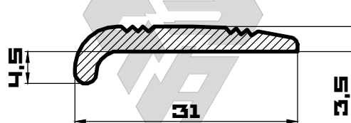
ИЗАР-А002 m=279 (гp/n.m)
